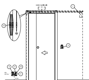
Esempio installazione su esistente Example of installation on existing frame
